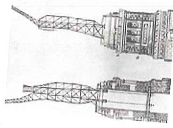
L'armature de la statue selon des plans de 1885.
